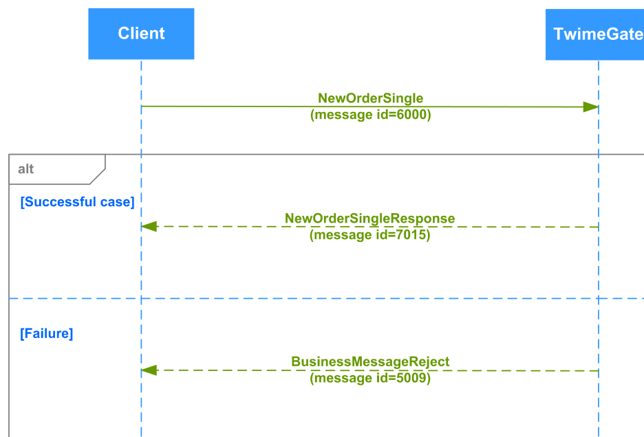
Рис. 17. Диаграмма. Добавление заявки с TimeInForce=0(Day)
