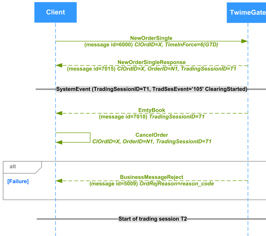
Рис. 16. Диаграмма. Отклонение многодневных заявок в клиринг
