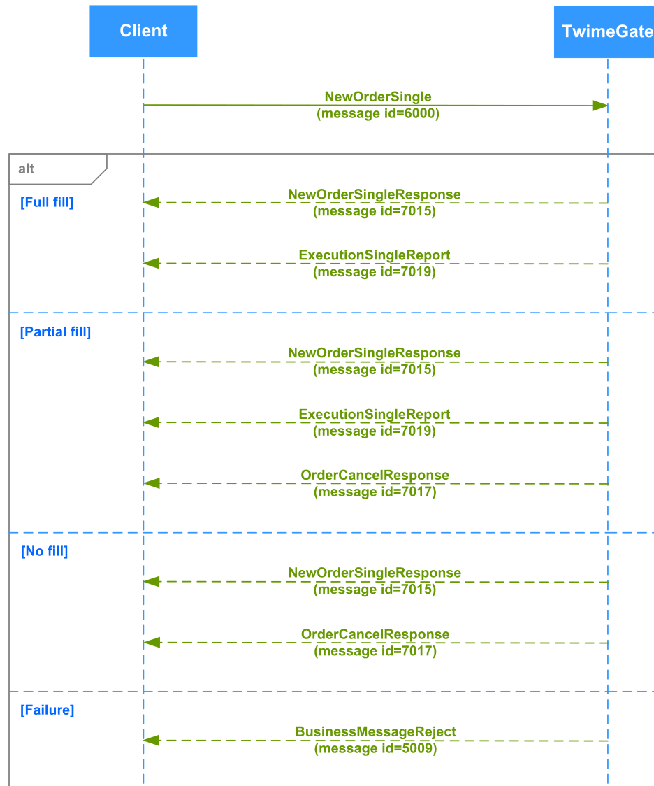
Рис. 18. Диаграмма. Добавление заявки с TimeInForce=3(IOC)
