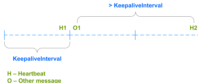
Рис. 3. Диаграмма. Отправка Heartbeat-сообщений от TwimeGate
