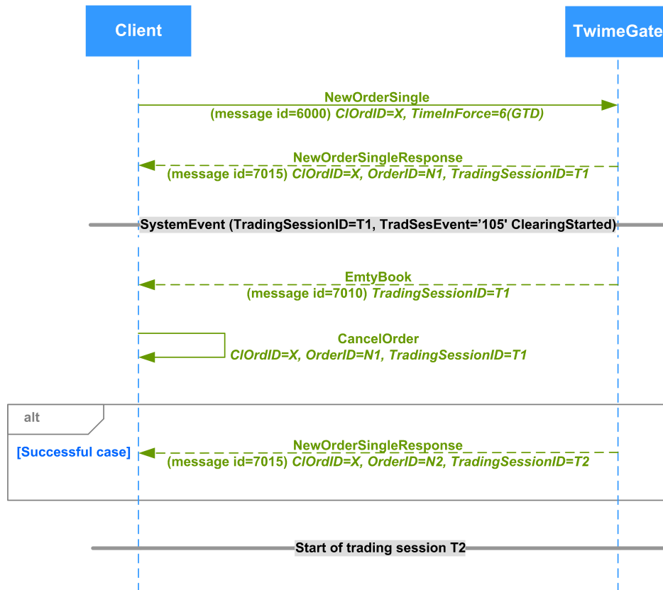
Рис. 40. Диаграмма. Перевыставление многодневных заявок
