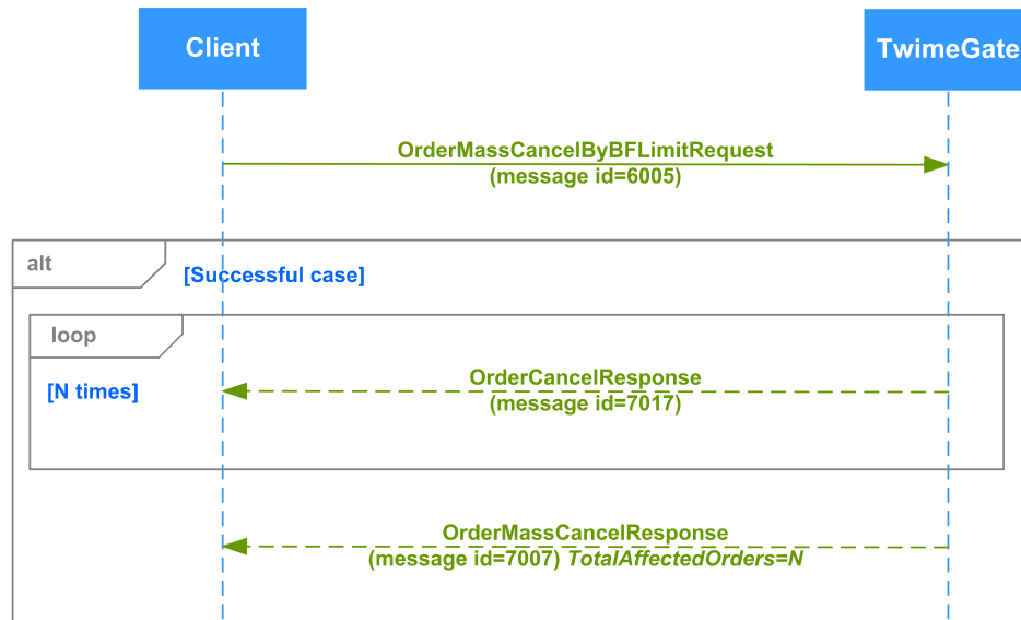
Рис. 41. Диаграмма. Запрос НКЦ на проверку достаточности обеспечения по БФ
