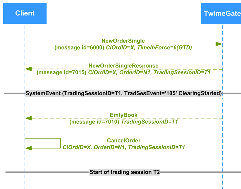
Рис. 38. Диаграмма. Очистка заявок на стороне клиента
