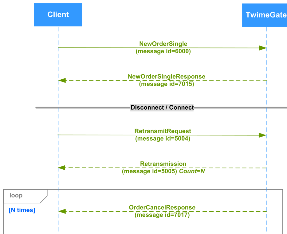
Рис. 39. Диаграмма. Автоматическое снятие заявок
