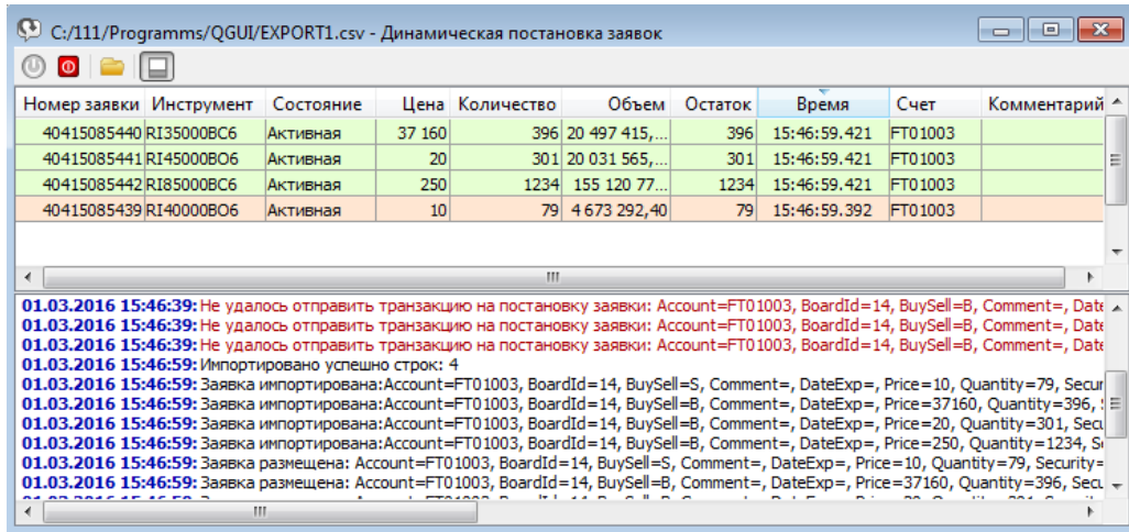
Рис. 6.48. Динамическая постанoвка заявок
