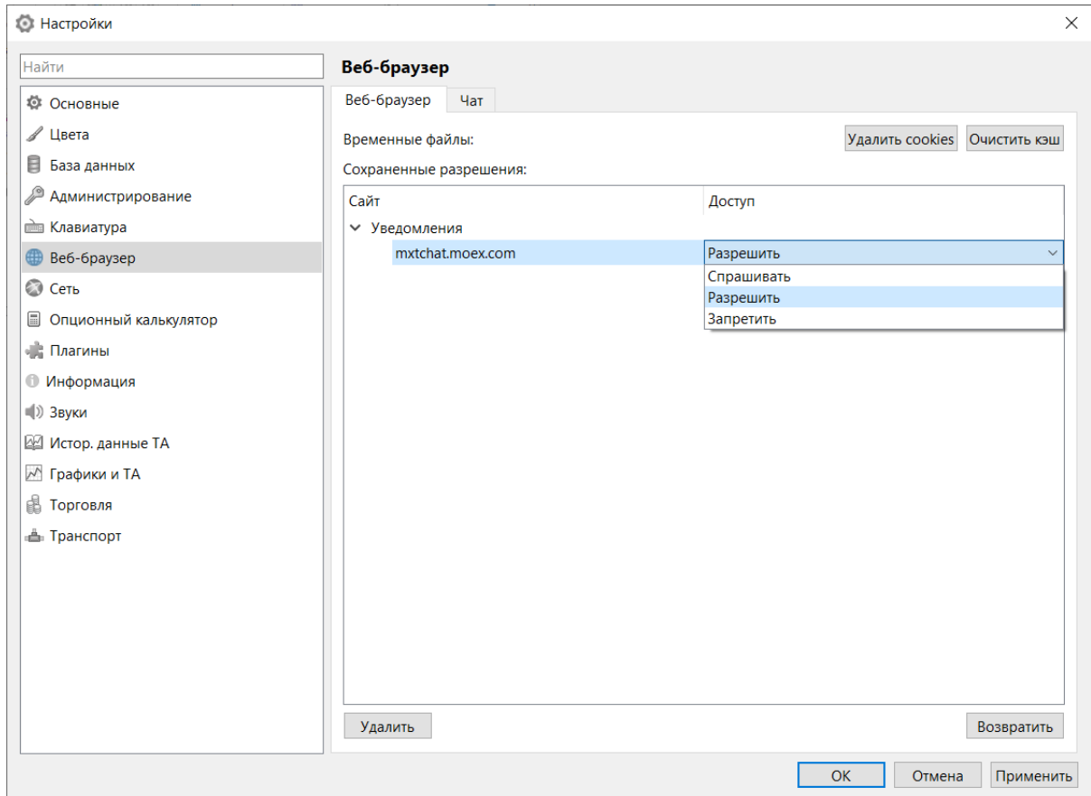
Рис. 10.11. Настройка веб-браузера
