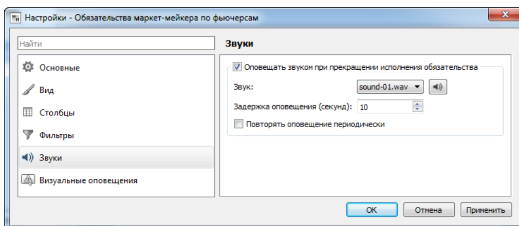
Рис. 8.6. Настройка звукового оповещения при неисполнении обязательств маркет-мейкера
