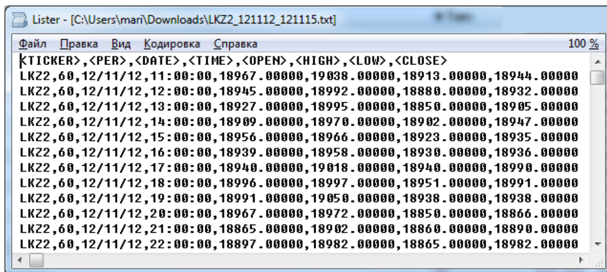
Рис. 9.41. Структура данных в экспортном файле
