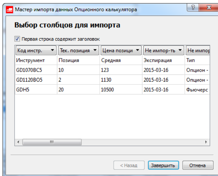
Рис. 7.13. Мастер импорта данных. Все обязательные данные выбраны.
