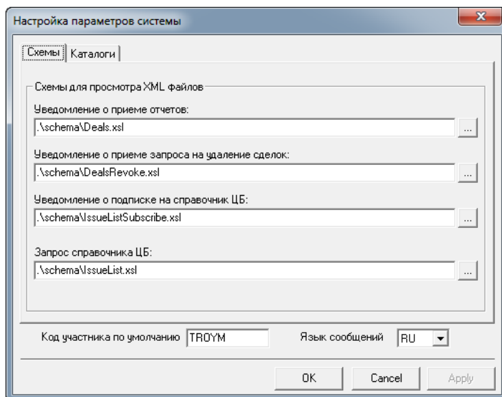
Рис. 4.14. Настройка схем для просмотра XML файлов
