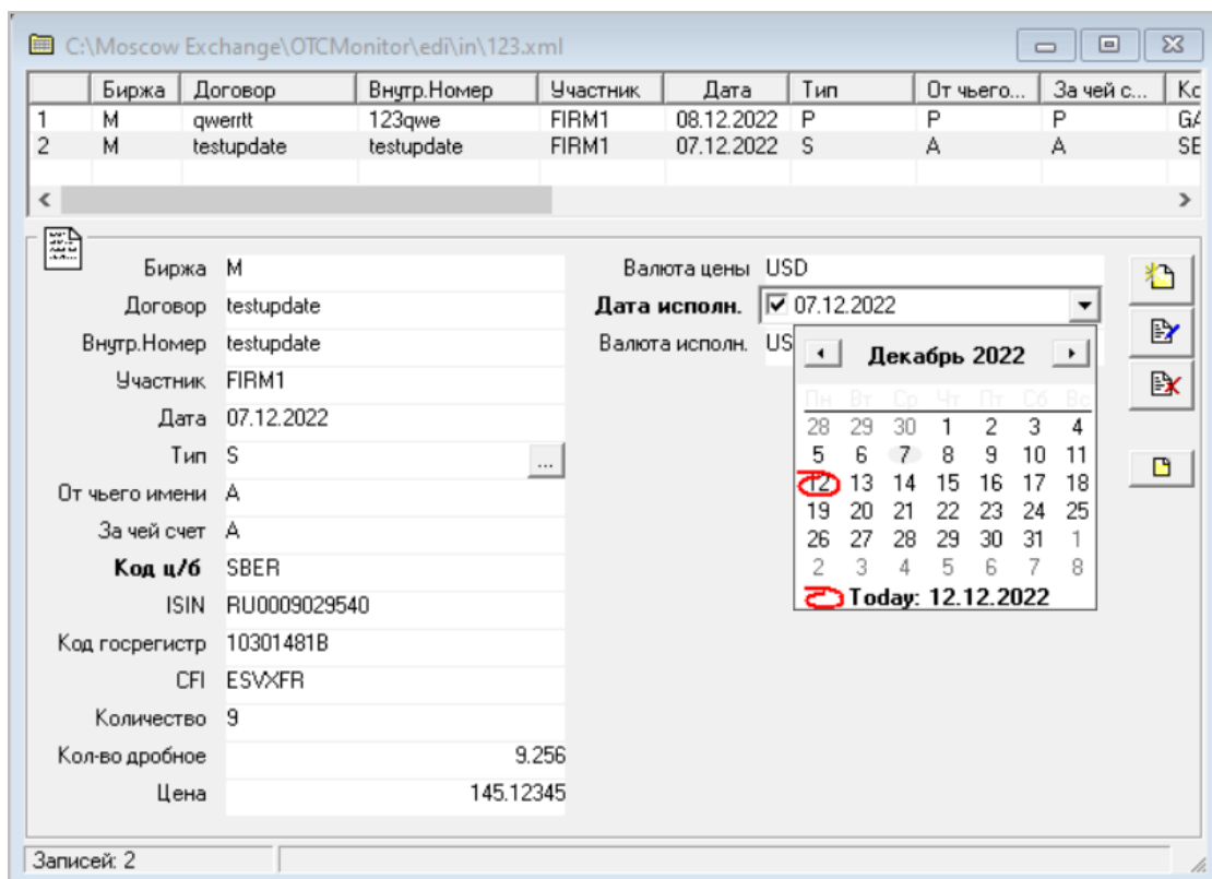
Рис. 4.1. Окно формирования отчета
