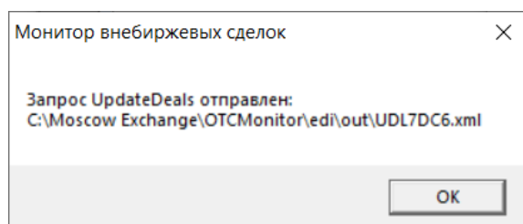
Рис. 4.4. Информационное окно
