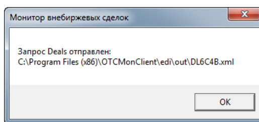
Рис. 4.5. Отправка отчета
