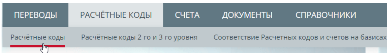
Рисунок 5-2 Меню программы
