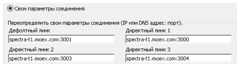
Рис. 13. Секция пользовательских настроек подключения
